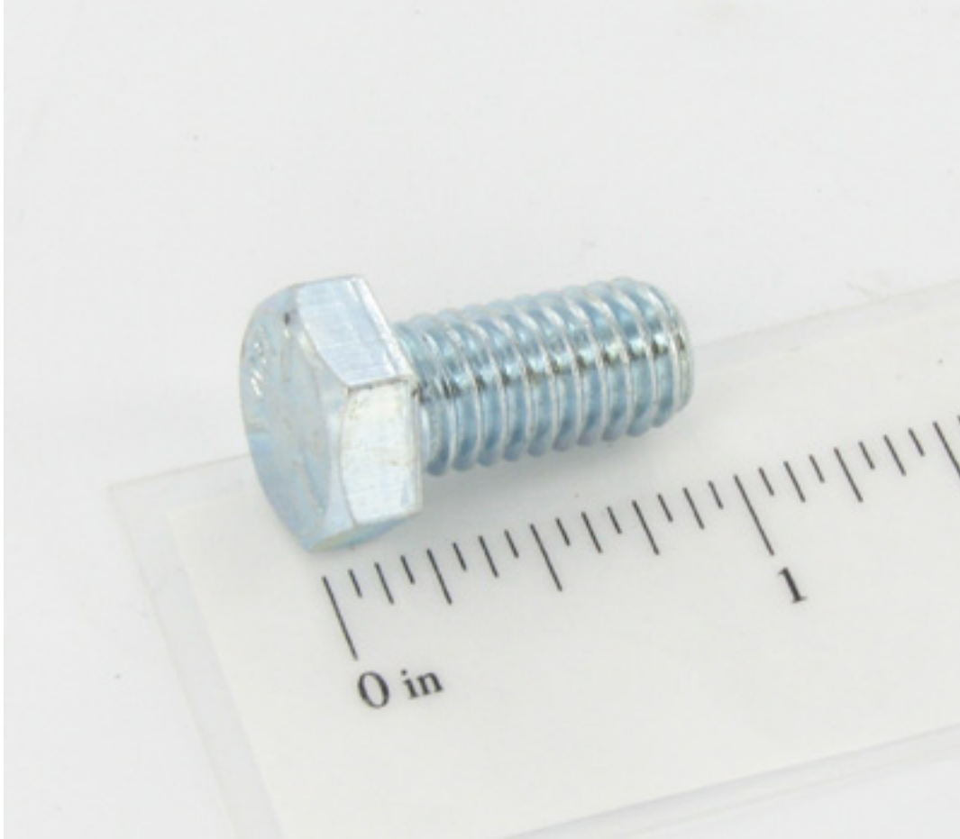
1/4-20ncx3/4lg hhcs
