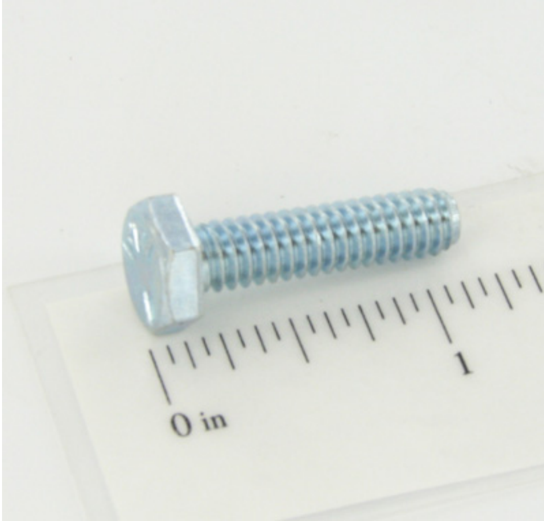
1/4-20ncx1lg hhcs
