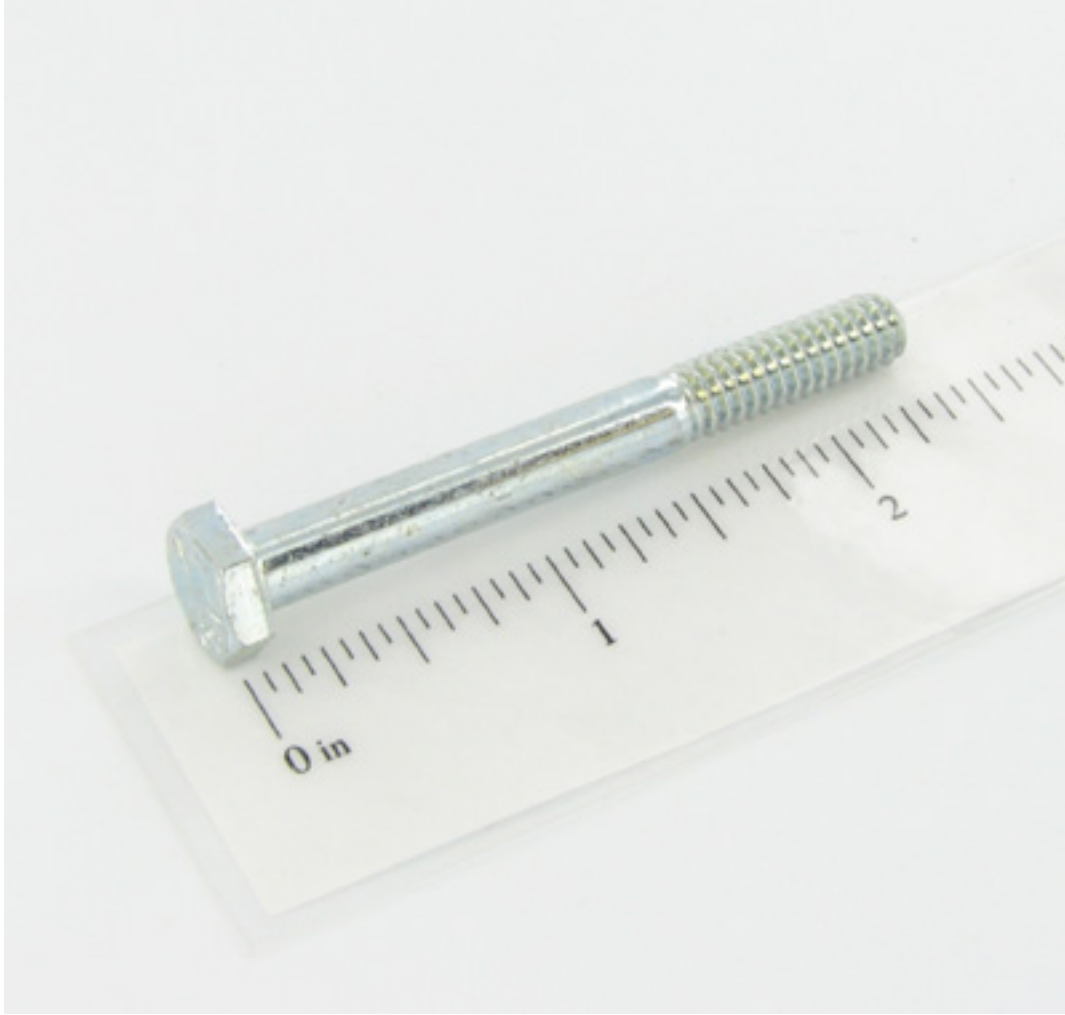
1/4-20ncx2-1/4lg hhcs
