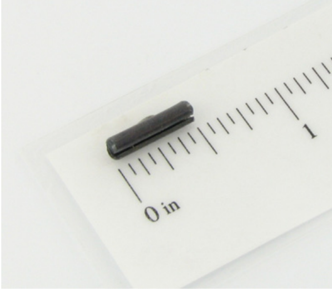
1/8diax1/2lg roll pin
