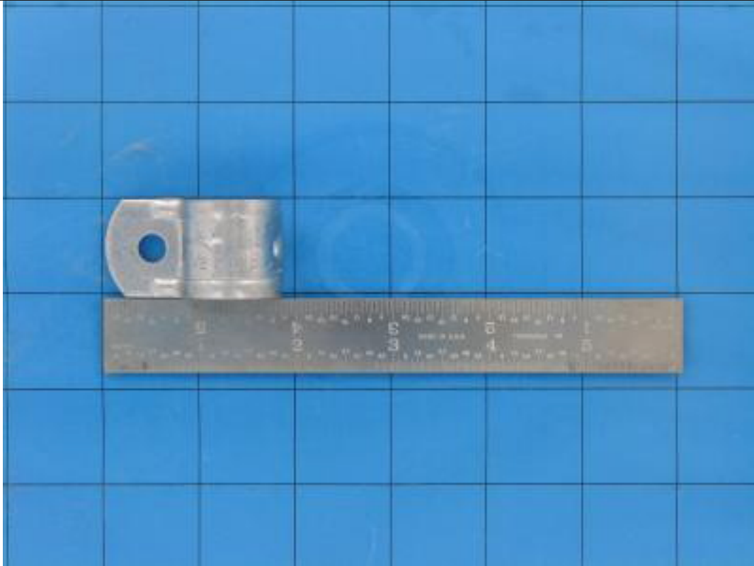
1/2" rmc conduit clamp
